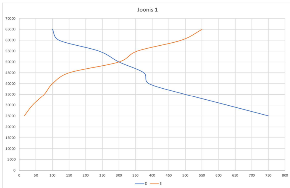
Joonis 1. SWI jäätmeenergia muunduri nõudlus ja pakkumine
